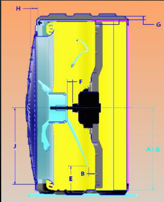
Optimize Edilmiş Hava Kanalı
